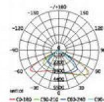
courbe de distribution de la lumière 100W
